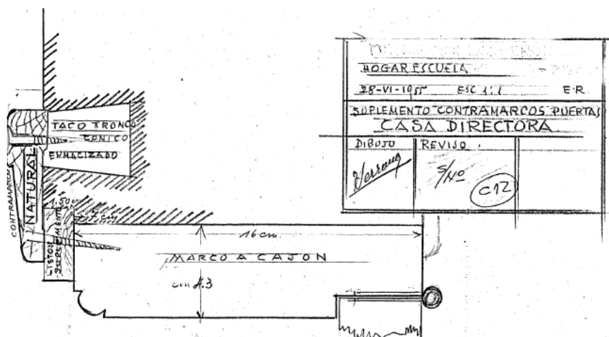
5. Plano 16228 Encadenado vigas-sección G de fecha 28/08/1950- Fondo documental del Museo.
